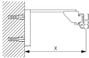
Smart Fix SG 11200 - SG 11205 e supporto SG 3603: Necessaria vite SG 10492 (M4x8).
