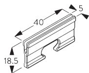
SG 10157 Spessore profilo incasso
