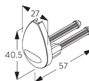
SG 4944 Tappo balza per guide
