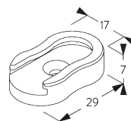
SG 10673 Base ferma-cavo guida doppio basso
