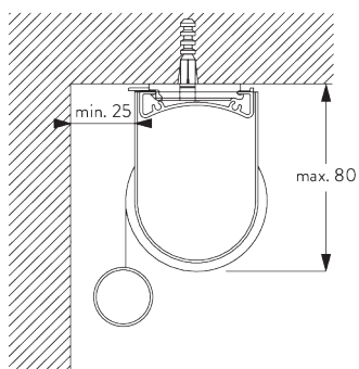
Barra portarullo SG 10534 e supporto click SG 10539
