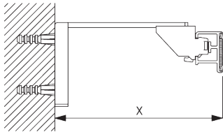
Smart Fix SG 11200 - SG 11205 e supporto SG 3603: Necessaria vite SG 10492 (M4x8).
