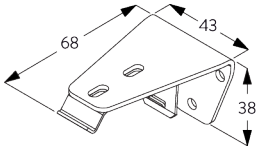
SG 2363 Supporto universale 68 mm
