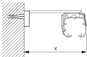
Smart Fix squadrato SG 11210 - SG 11215 e supporto SG 2302: Necessaria vite SG 10395 (M4x6).
