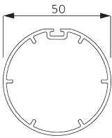
SG 2352 Profilo ø 50 mm
