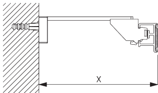
Smart Fix squadrato SG 11210 - SG 11215 e supporto SG 3603: Necessaria vite SG 10492 (M4x8).
