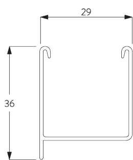
SG 8301 Profilo
